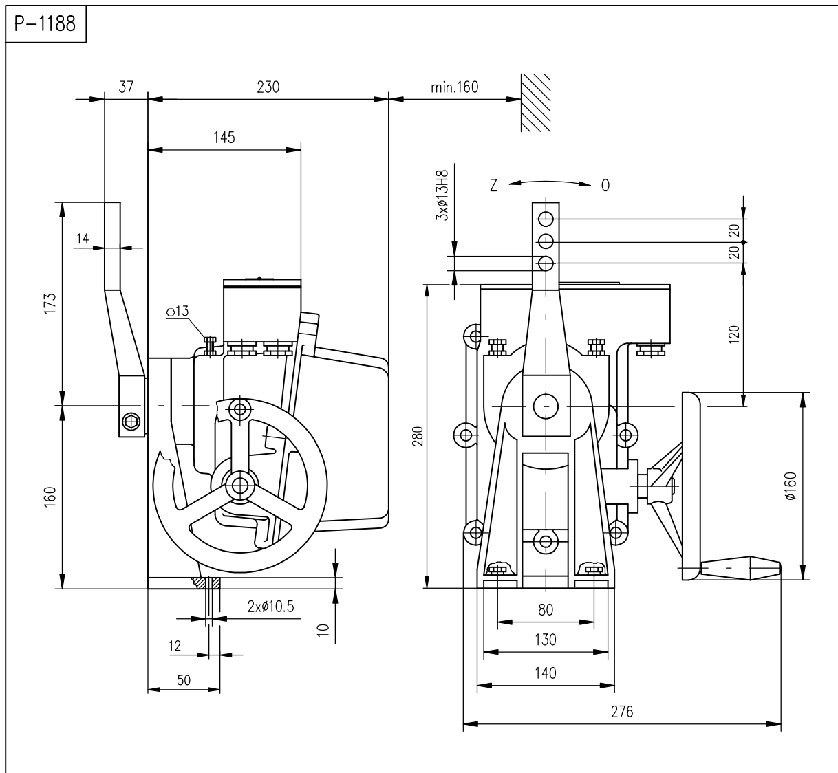
Rozmerový náčrtok SP 1-Ex – vyhotovenie so stojanom a pákou
