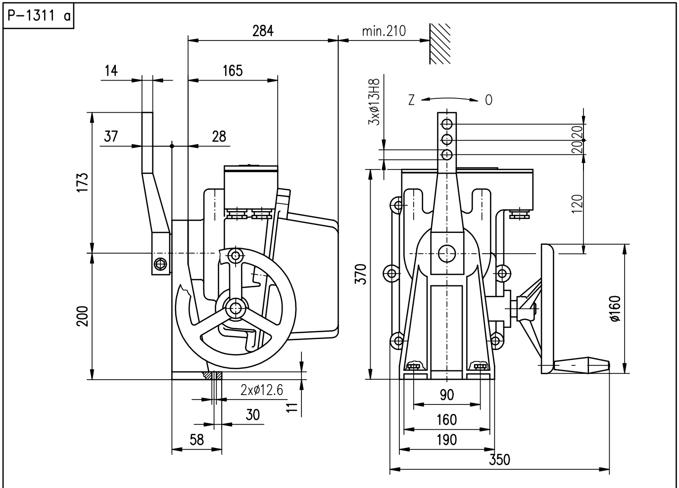
Rozmerový náčrtok – pákové vyhotovenie pre ES SP 2-Ex P-1311 Stožan + páka
